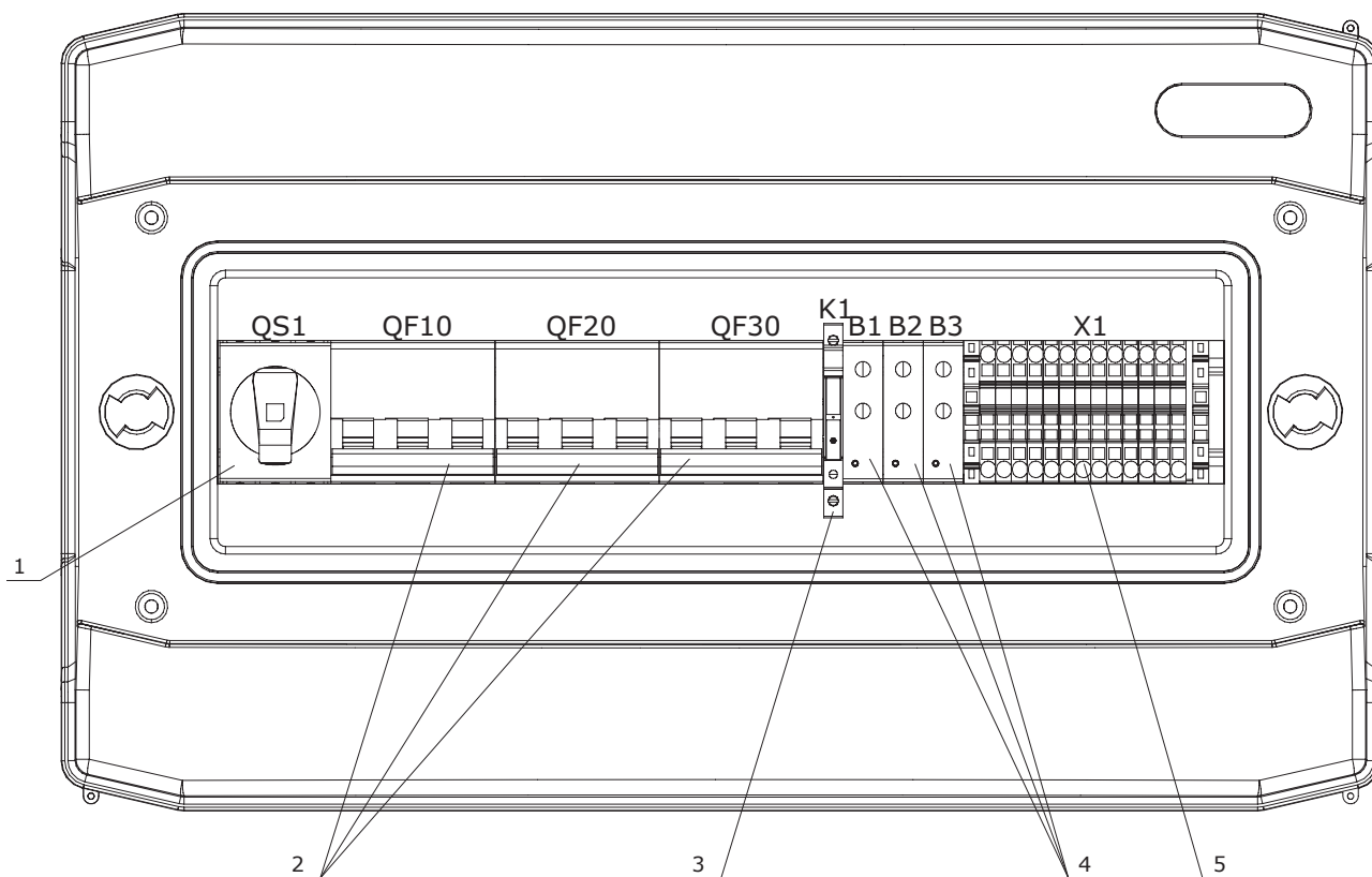
Рис. 9 Распределительный шкаф
