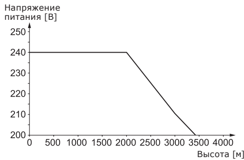
Рис. 18 Напряжение питания для однофазного электродвигателя в зависимости от высоты над уровнем моря.
