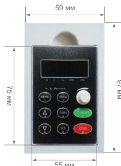
Модель FCI-KP-S 3,7 - 7,5 кВт LED панель
