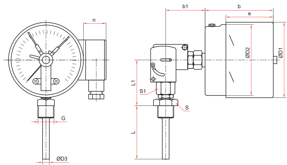
Универсальное присоединение
