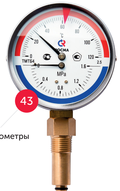
Термометры общетехнические с защитной латунной гильзой
