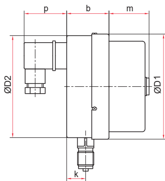
Радиальное присоединение
