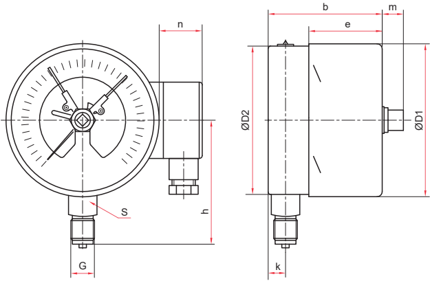
Радiallyное присоединение
