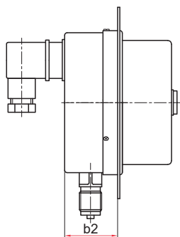
Радиальное присоединение с передним фланцем
