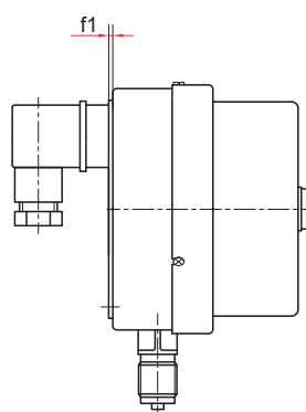
Радиальное присоединение с задним фланцем
