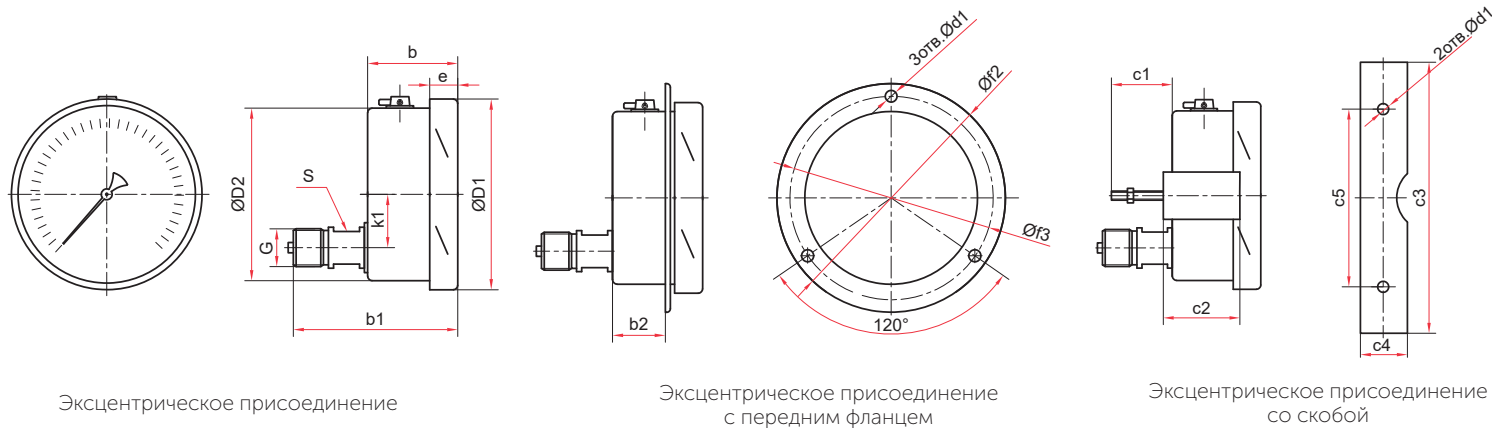
Основные размеры (мм), вес (кг), объем (мл)
