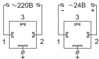
Схема подключения катушки
