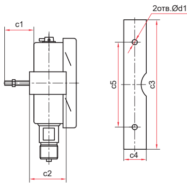
Радиальное присоединение со скобой
