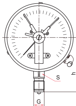
Радиальное присоединение (100 МПа)
