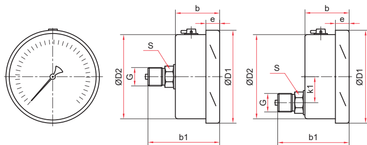
Осевое и эксцентрическое присоединения (Ø100 мм)
