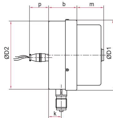
Радиальное присоединение (100 МПа)
