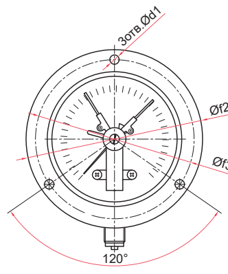
Радиальное присоединение с передним фланцем (100 МПа)
