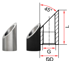
Для термометров БТ №20, №21
