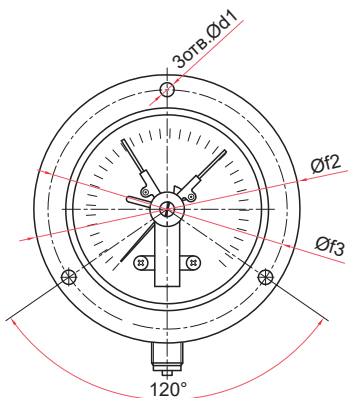
Радиальное присоединение с передним фланцем
