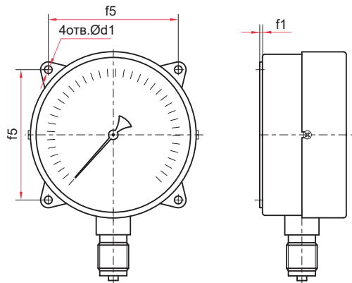
Радиальное присоединение с задним фланцем (Ø100, 150, 160 мм)
