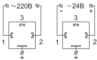
Схема подключения катушки
