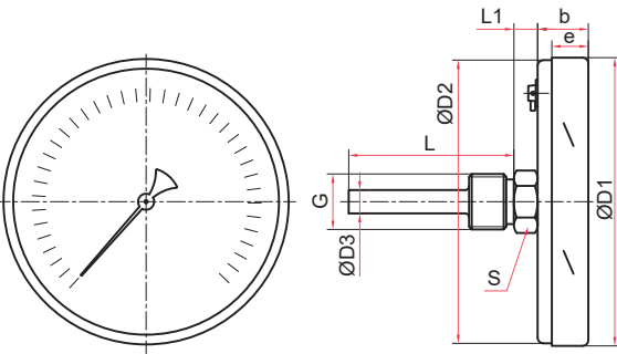
Осевое присоединение
