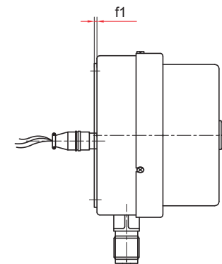
Радиальное присоединение с задним фланцем (100 МПа)
