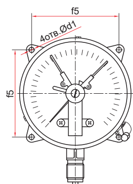
Радиальное присоединение с задним фланцем
