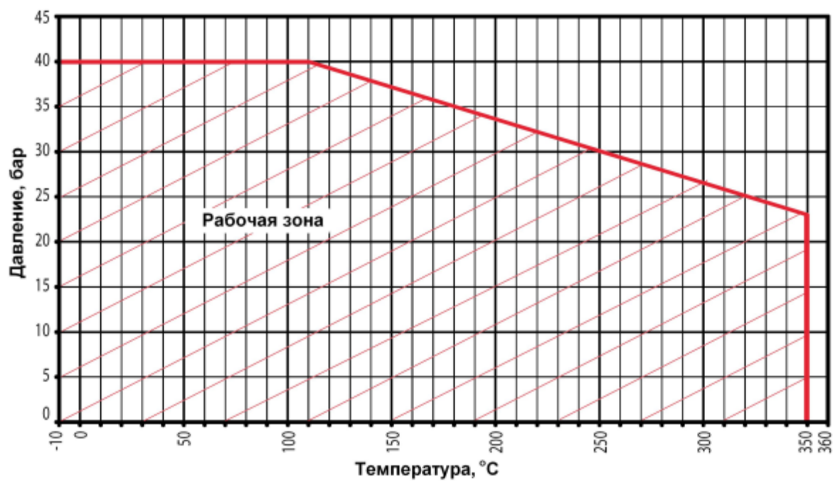
Диаграмма Температура-Давление
