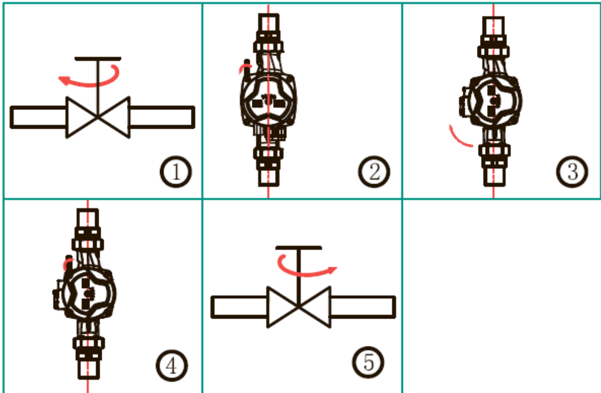
Рис.3. Последовательность установки головной части насоса.
