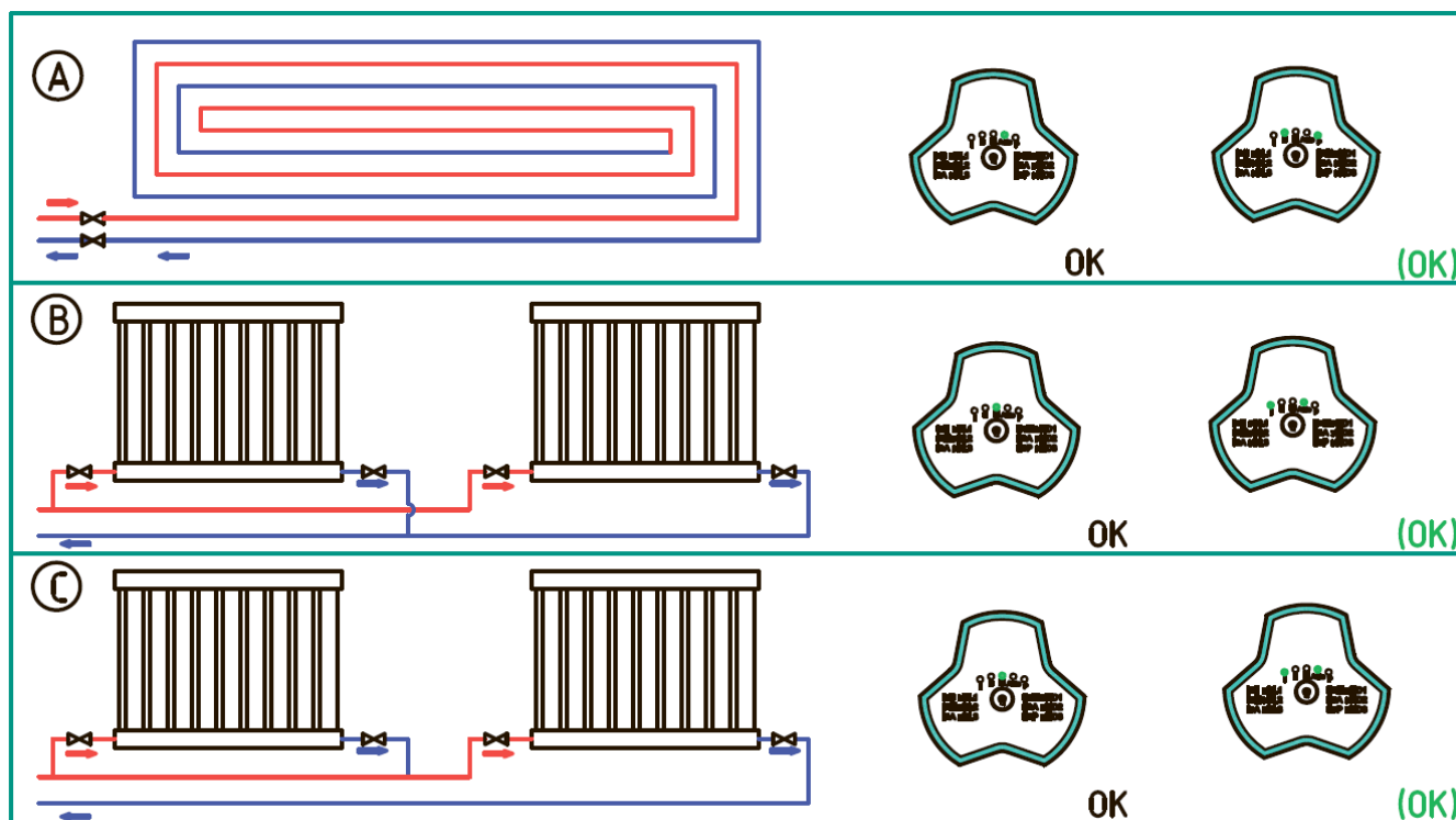
Рис.8 Система отопления
