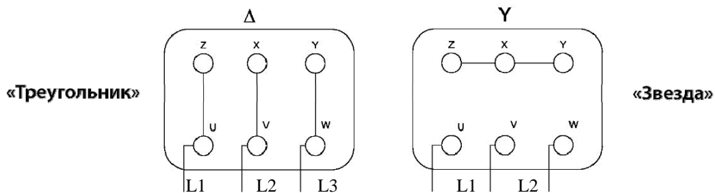
Схемы подключения: «треугольник» и «звезда»
