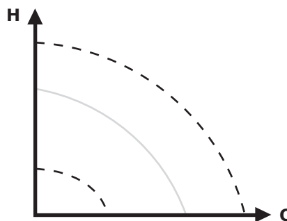
Рис. 53 Режим эксплуатации в соответствии с постоянной характеристикой
