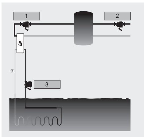
Рис. 43 Функциональная схема системы отопления на основе использования теплоты грунта
