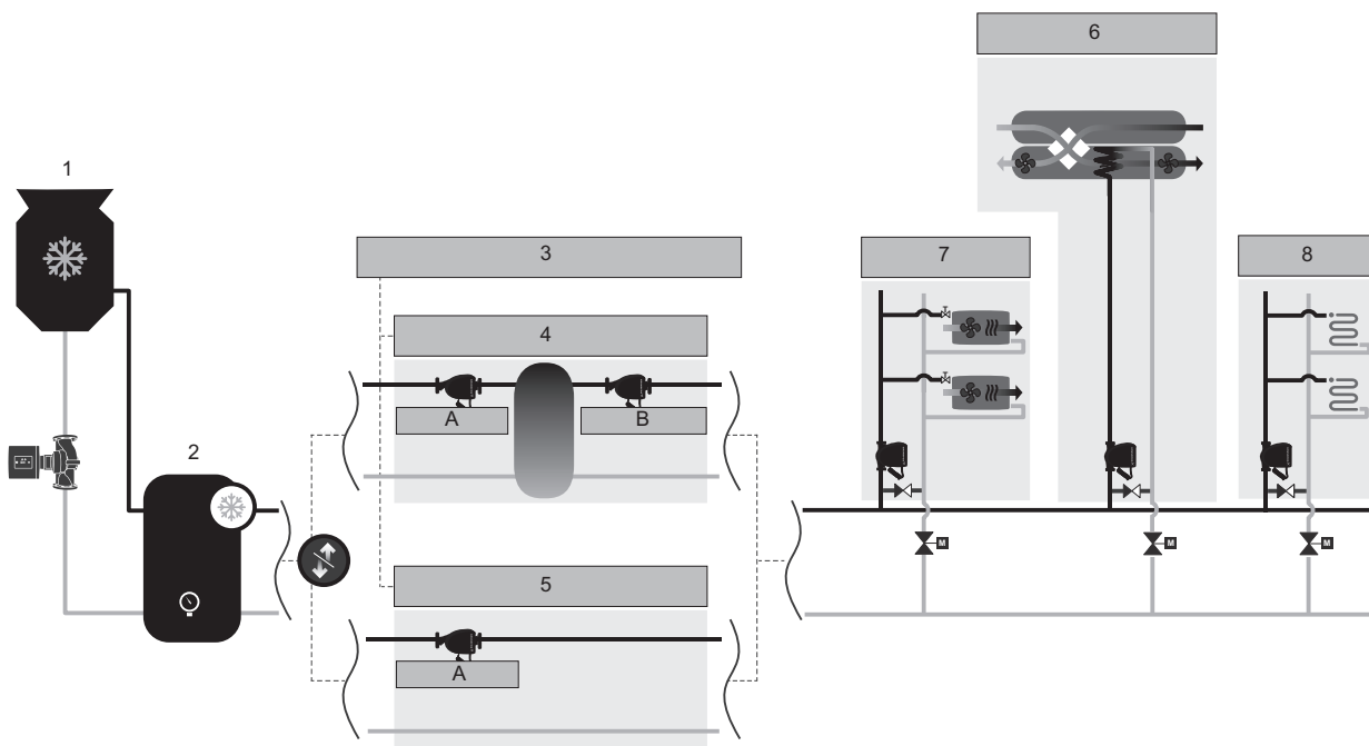
Рис. 42 Функциональная схема системы охлаждения в коммерческом здании
