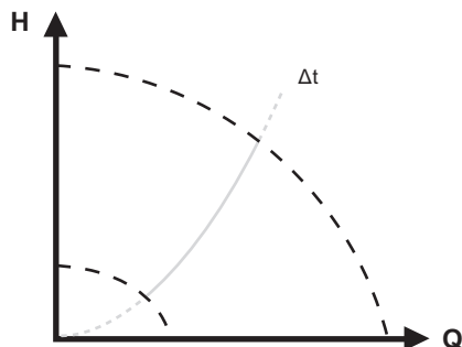
Рис. 51 Перепад температур
