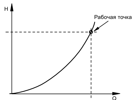
Рис. 1 Характеристика системы
