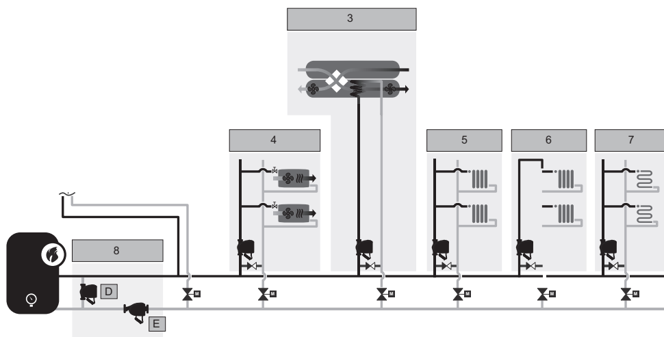
Рис. 41 Функциональная схема системы отопления в коммерческом здании
