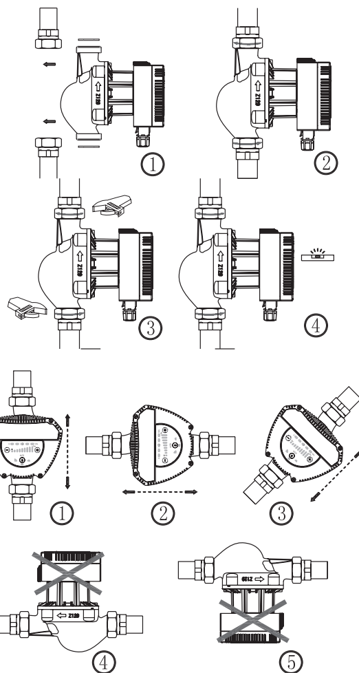
Рис. 33 Варианты монтажа
