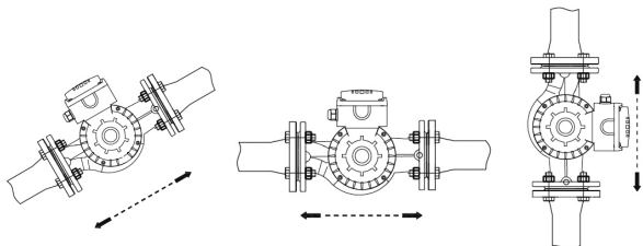
Рис. 56 Варианты монтажа
