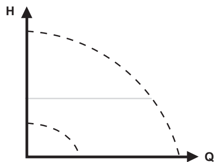
Рис. 47 Регулирование по постоянному давлению
