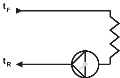
Рис. 50 Насос со встроенным датчиком
