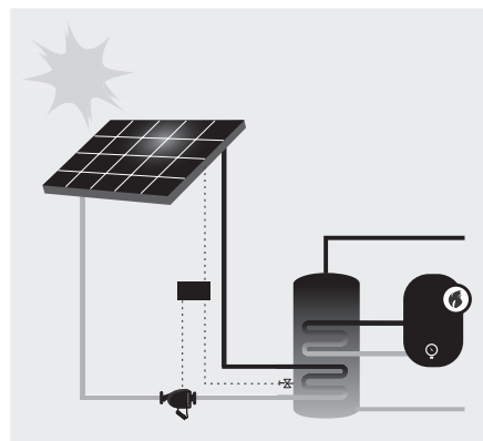
Рис. 44 Функциональная схема системы отопления на основе использования энергии солнца
