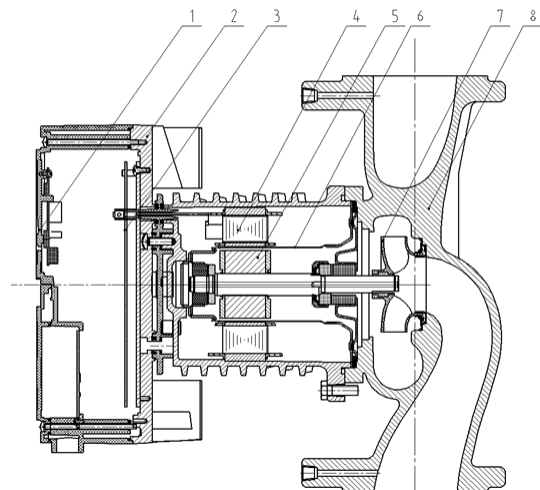
Рис. 55 Автоматический насос MEGA S
