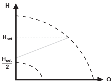
Рис. 46 Регулирование по пропорциональному давлению
