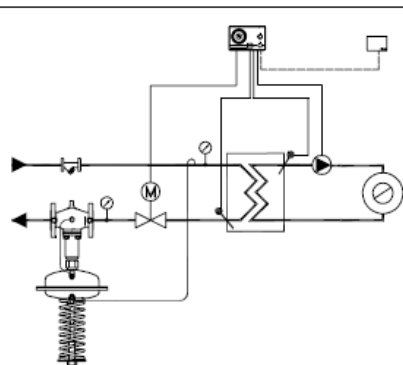
Регулятор перепада давлений AFPB/VFQ2 устанавливается только на обратном трубопроводе
